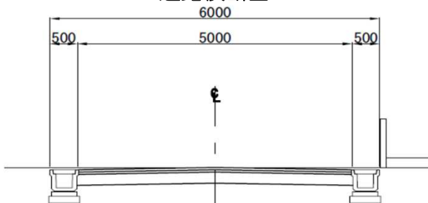
橋梁區間横断面
