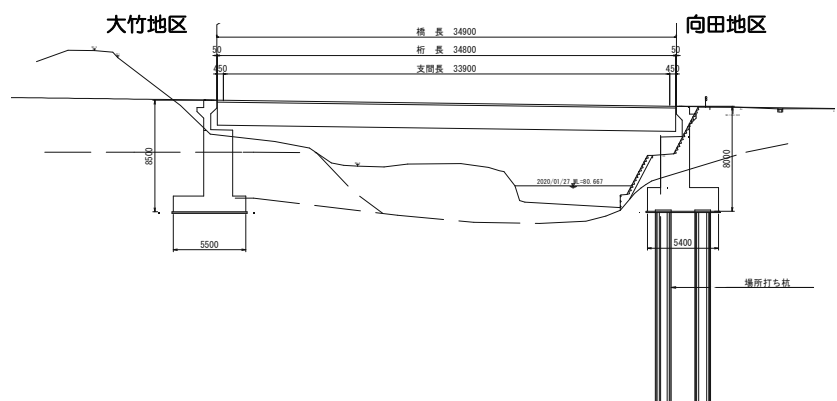
橋梁側面図
