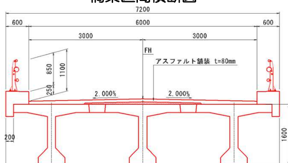
橋梁區間横断面
