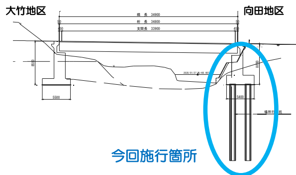
橋梁側面図
