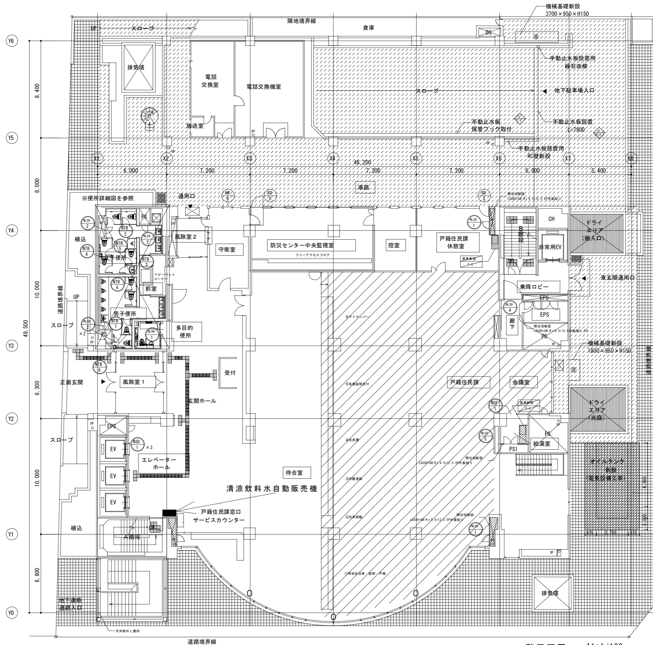
1階平面図
