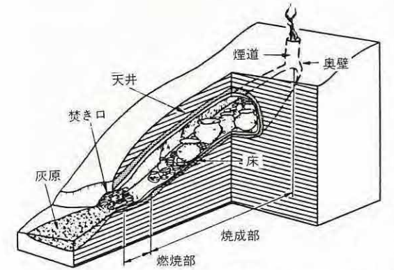
須恵器窯（地下式窖窯）の模式図
