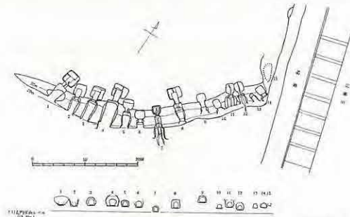
宗禅寺横穴墓群配置図
