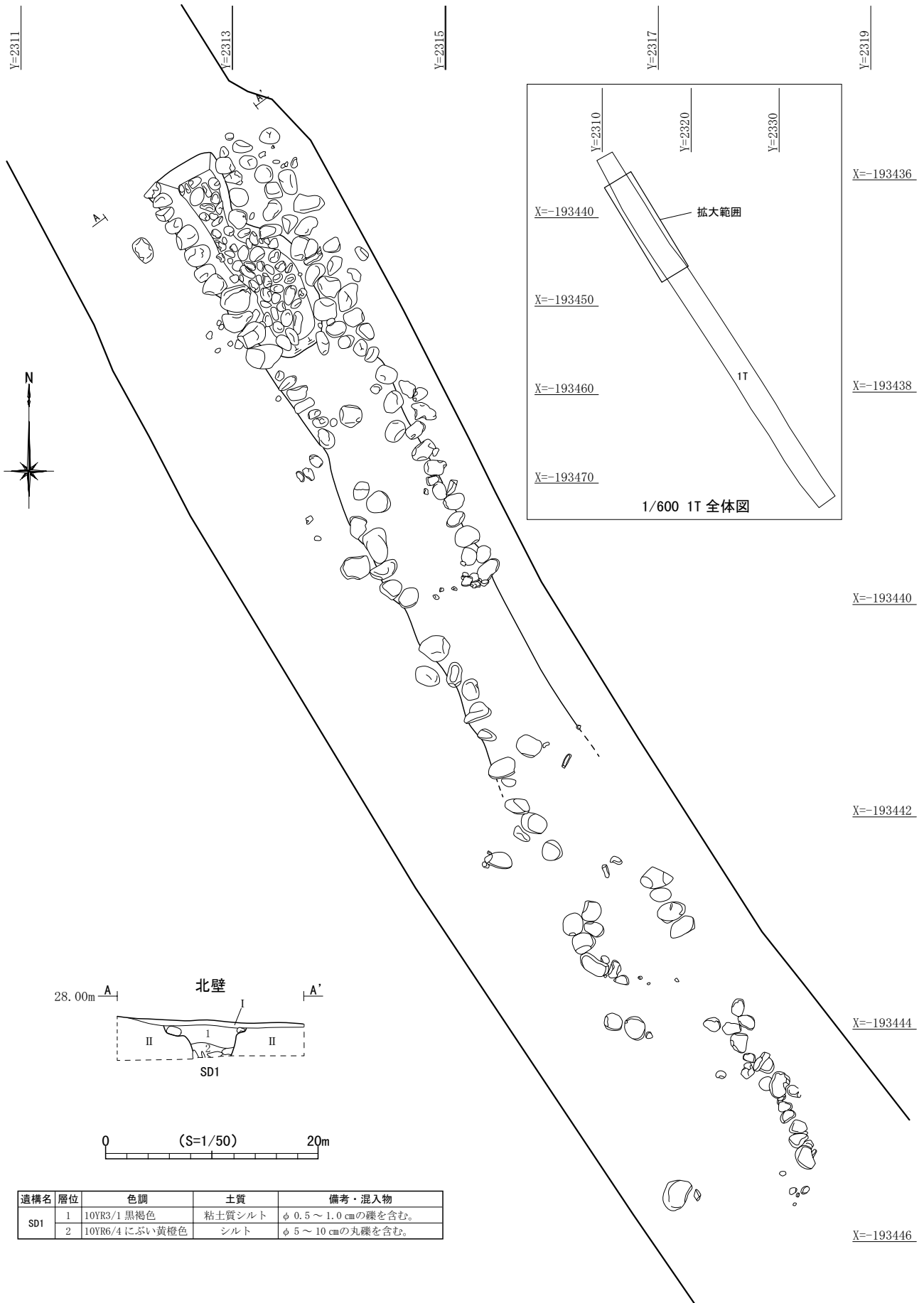
SD1 (溝跡) 平面図
