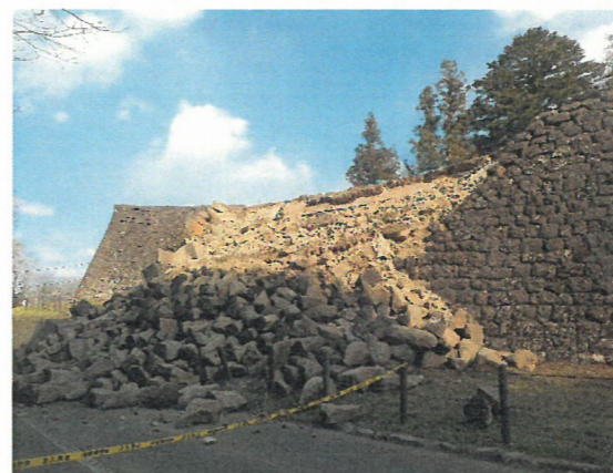
本丸北西石垣被災状況（南西から）
