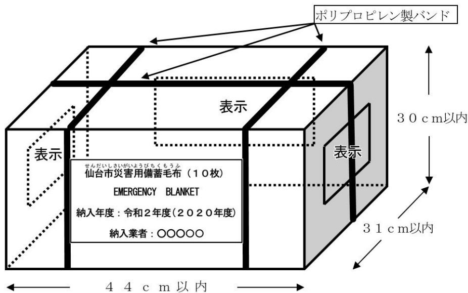
〈箱の外観図〉
