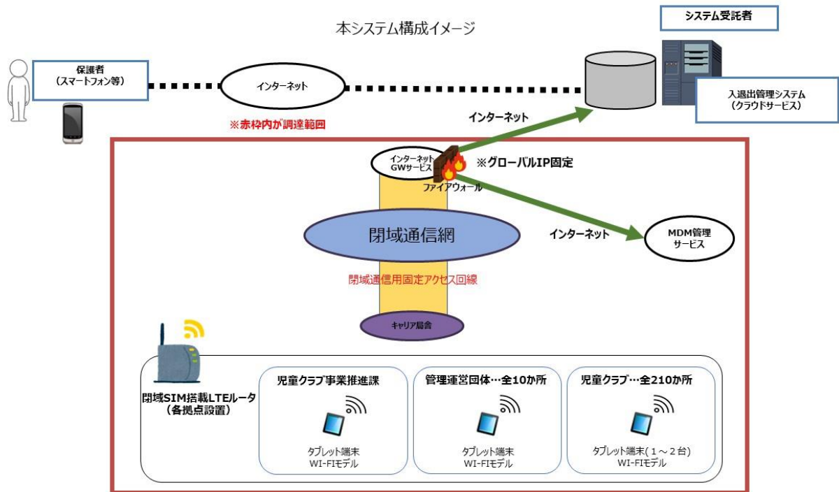
図2 児童クラブ業務支援システム構成イメージ
