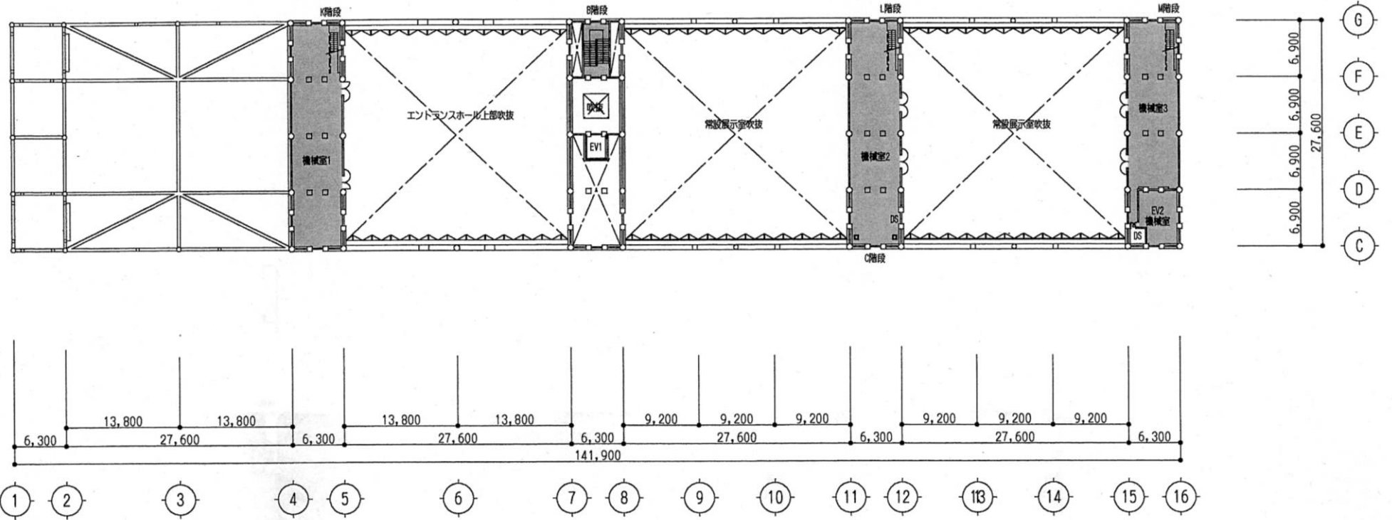
5階平面図
