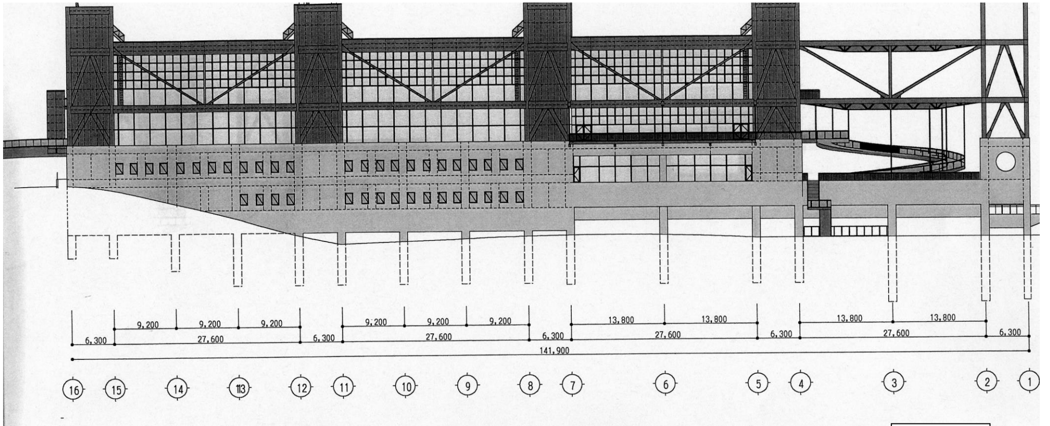
西立面图
