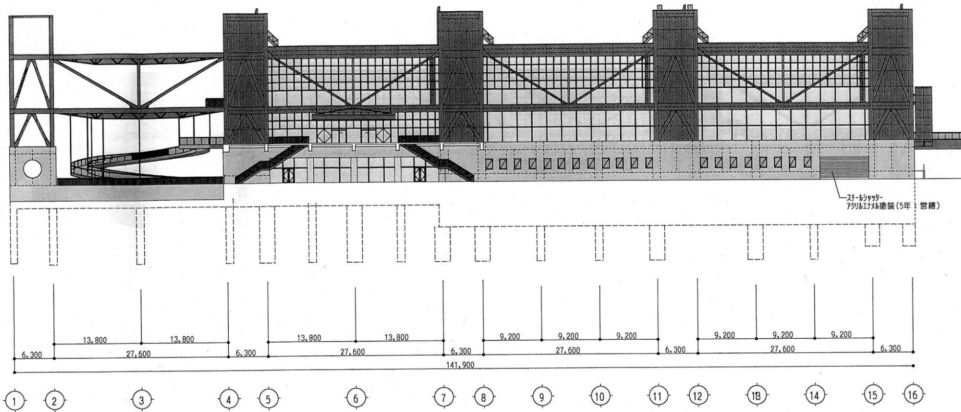
東立面図
