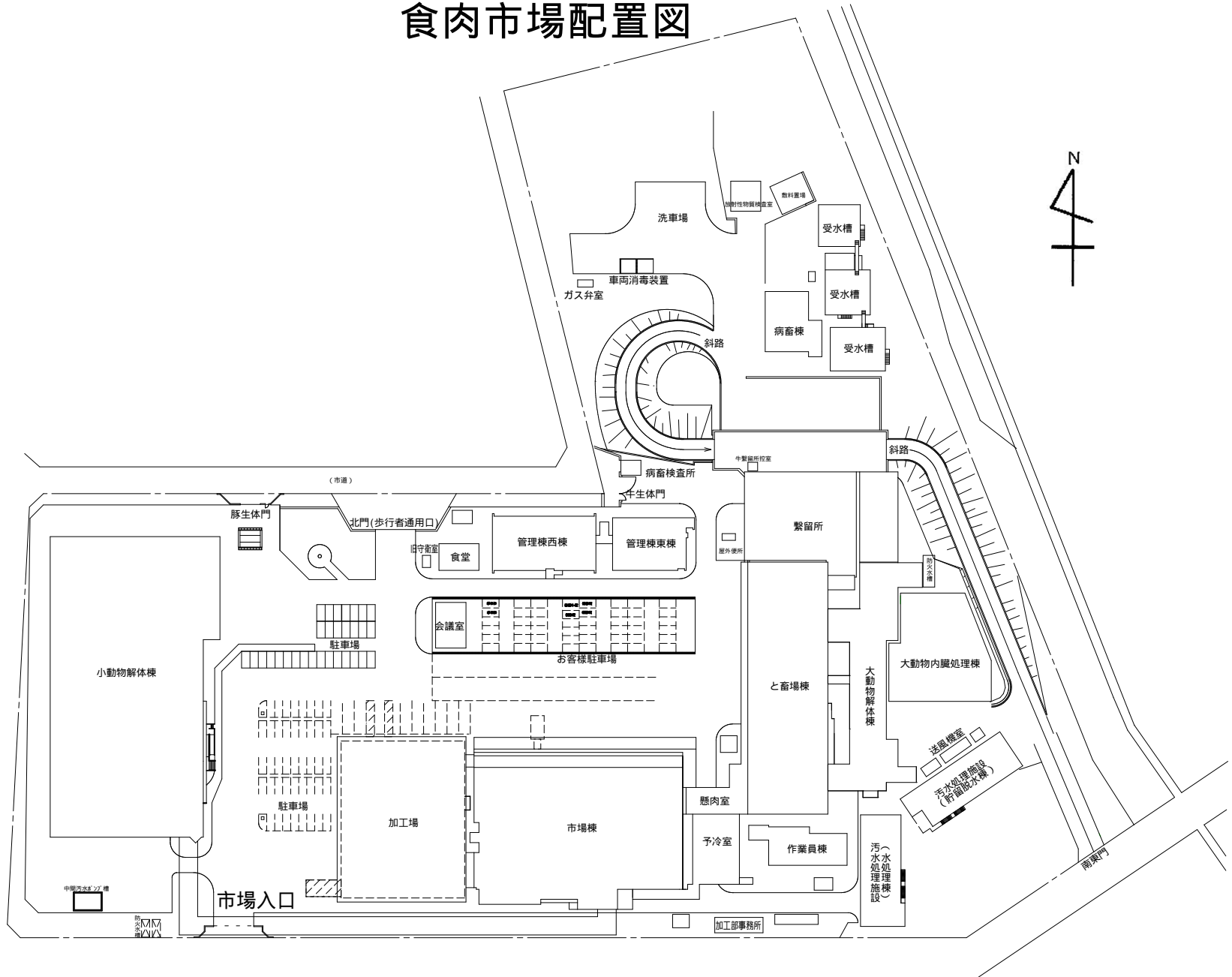
仙台市中央卸売市場食肉市場 配置図
