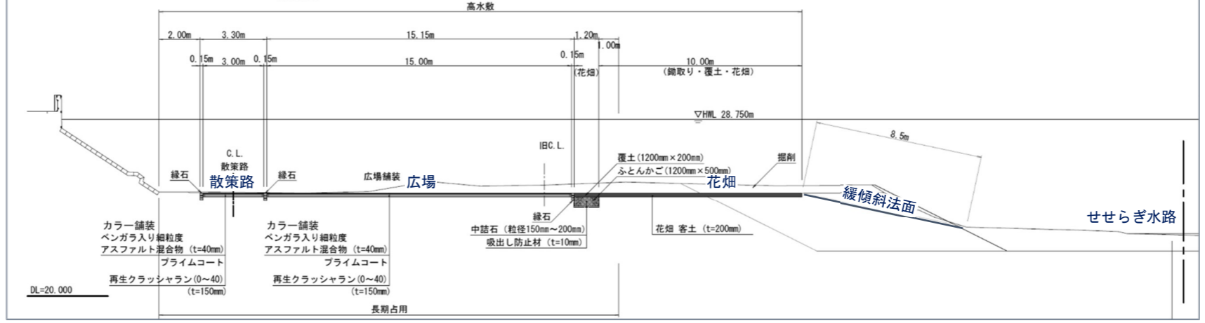
西公園側河川敷 標準断面図
