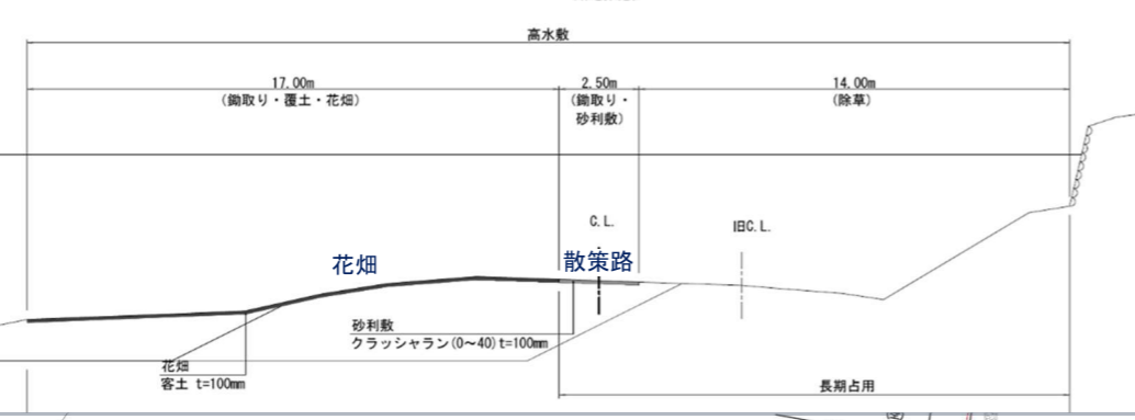
青葉山公園側河川敷 標準断面図
