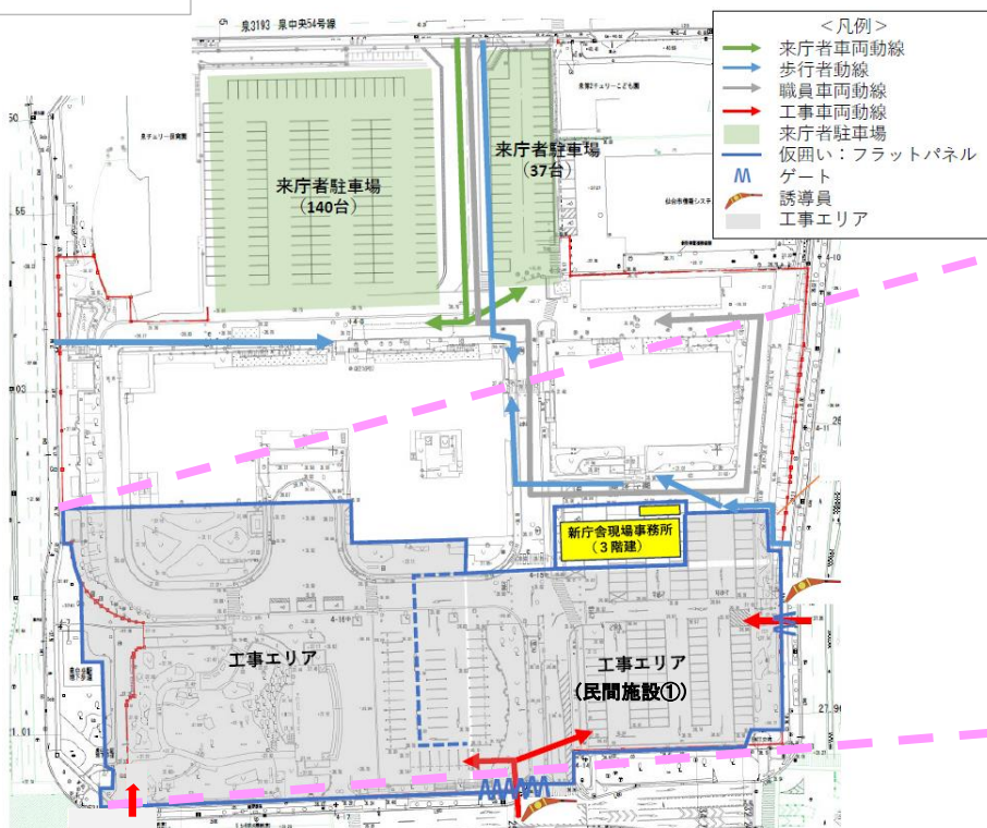
仮設計画図
