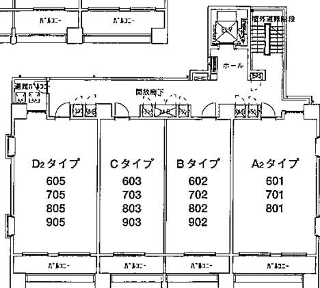
6階～9階平面図
