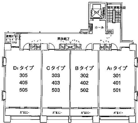
3階～5階平面図
