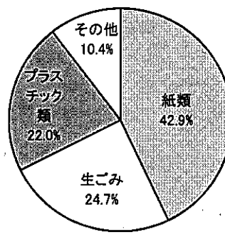
図 18 事業系可燃ごみの組成 (仙台市：平成 26 年度)
