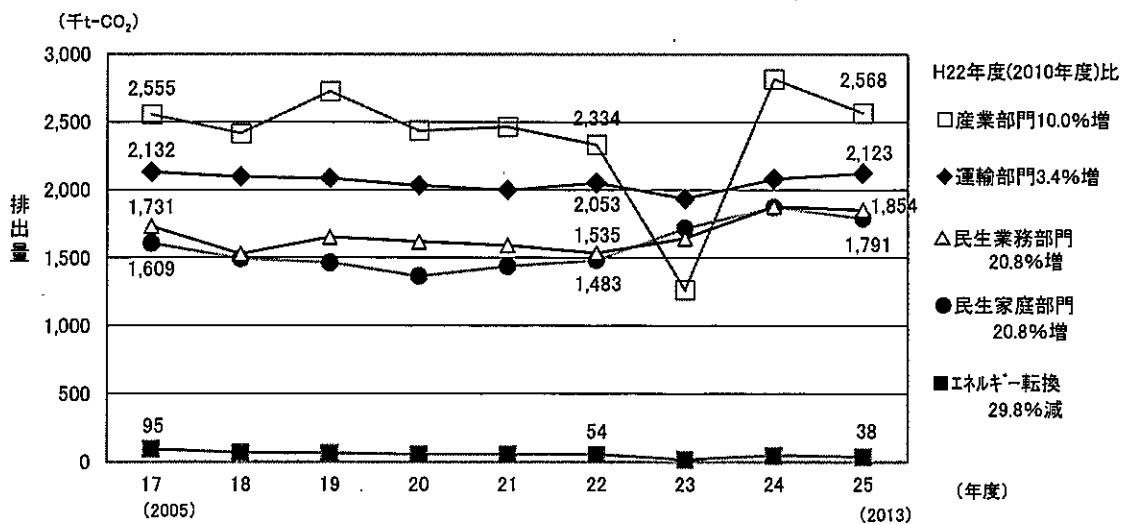
図9 二酸化炭素の部門別排出量の推移（仙台市）（エネルギー起源二酸化炭素）
