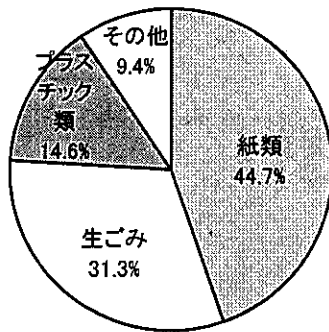
図 17 家庭ごみの組成 (仙台市：平成 26 年度)
