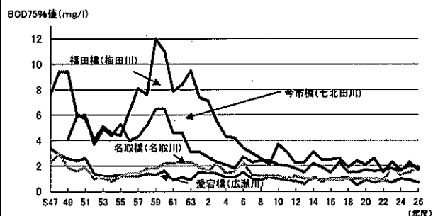
図 26 各河川におけるBODの経年変化(仙台市)
