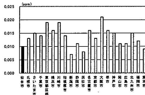
図 27 二酸化窒素濃度の大都市間比較(平成 25 年度)
