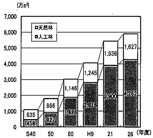
図 22 民有林材積の推移 (宮城県)
