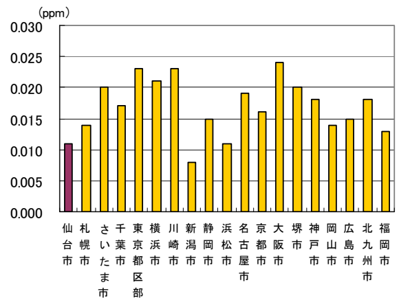
図26 二酸化窒素*濃度の大都市間比較（2008年度）
