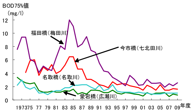
図25 各河川におけるBOD*の経年変化
