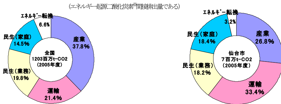
図7 全国と仙台市の部門別二酸化炭素排出量の比較 (2005年度)
