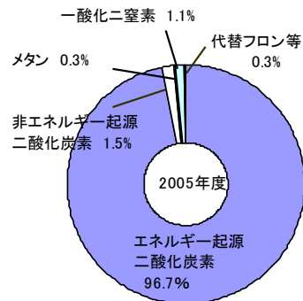
図6 温室効果ガスの構成
