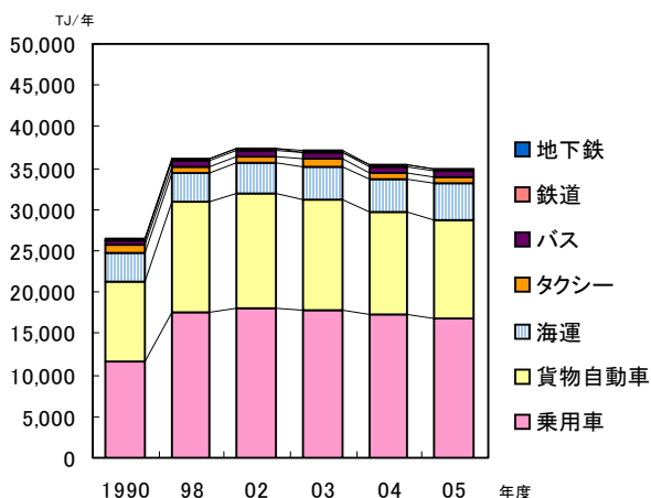
図9 運輸部門のエネルギー消費量の推移
