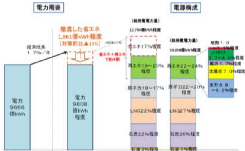
図1-6 2030 年度における電力需要及び電源構成
