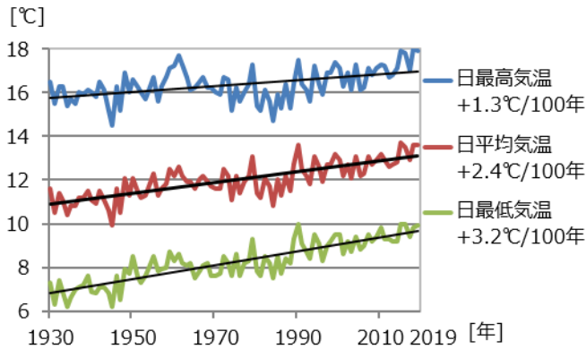
図1-7 年平均気温の長期変化傾向
