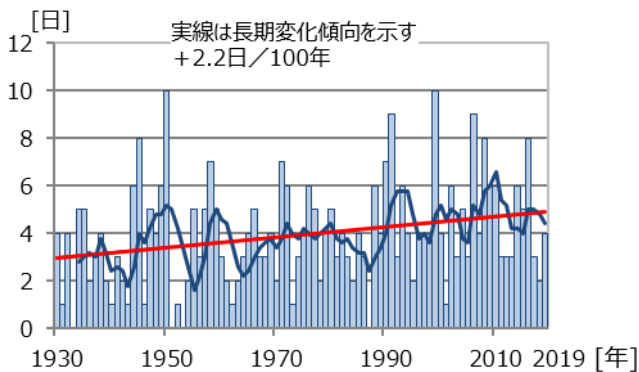
図1-9 日降水量50ミリ以上の年間日数の変化
