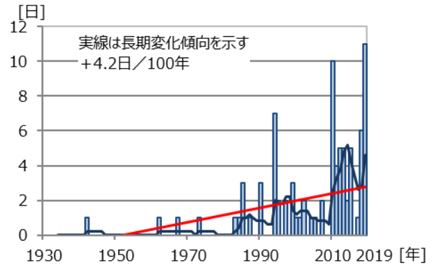
図1-8 熱帯夜日数の変化
