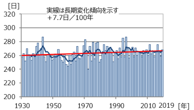
図1-10 無降水日数の変化
