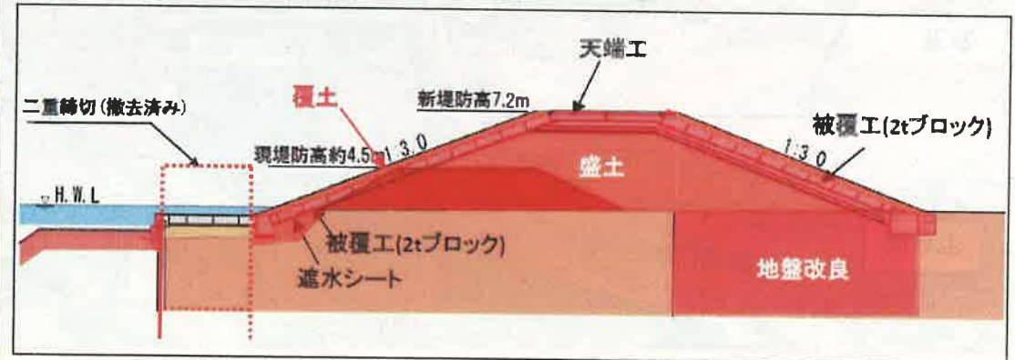
■ 河口部右岸堤防復旧断面図(閉上水門下流:地点①)
