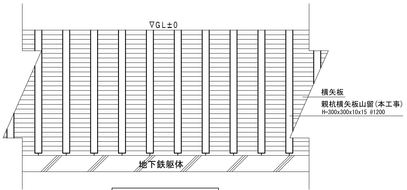
立面・展開図
