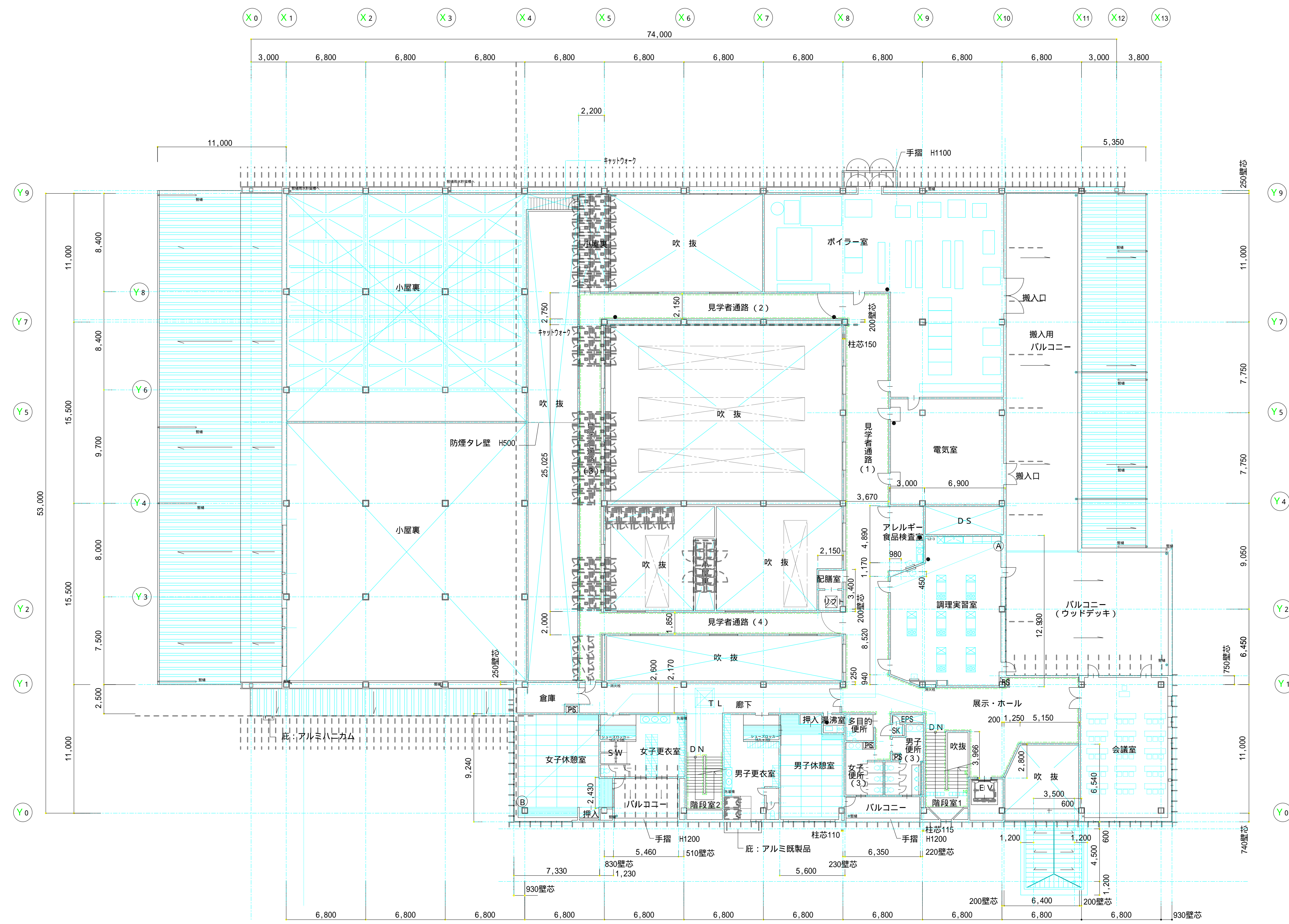
2階 平面図
