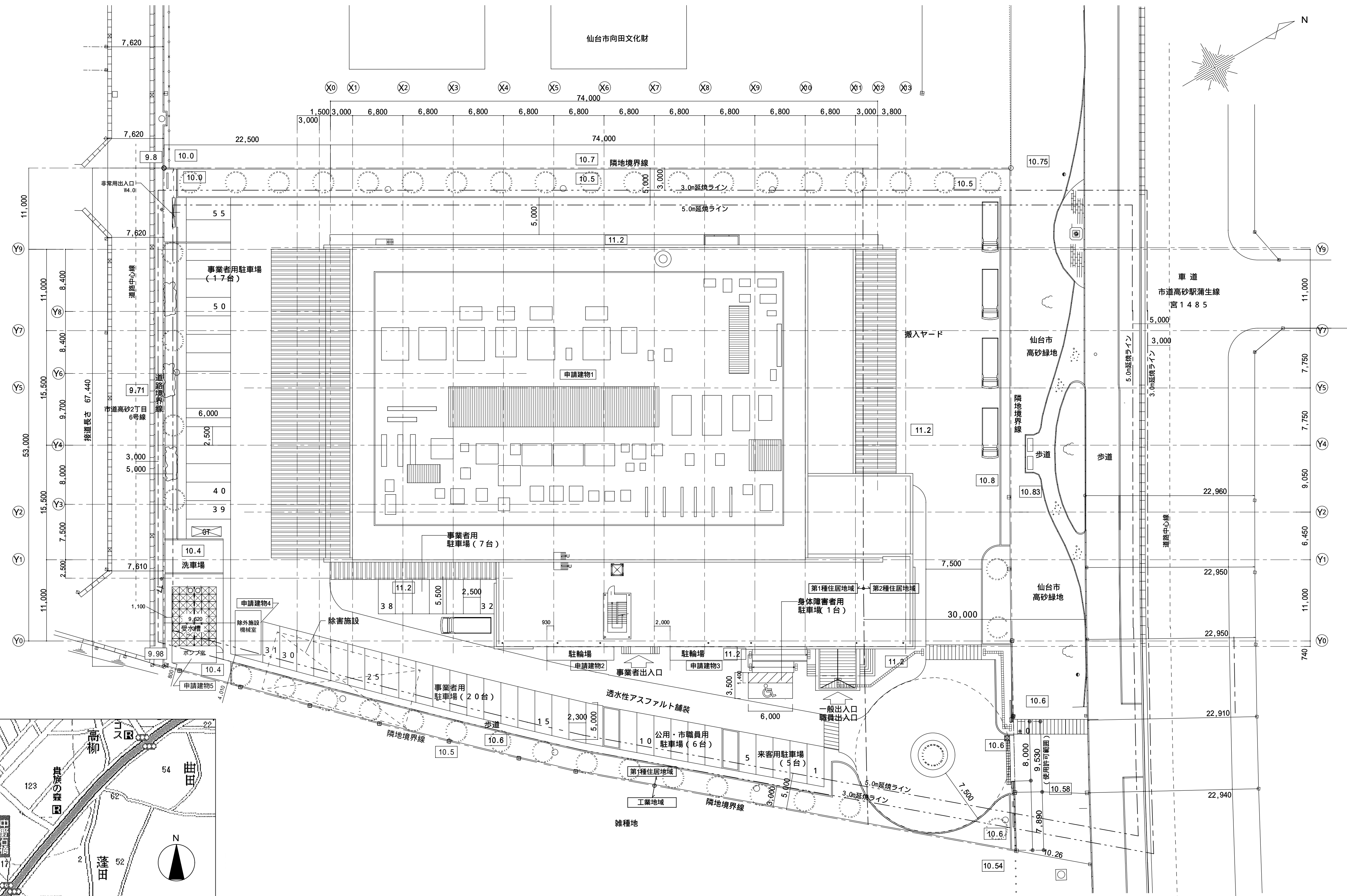
配置図 [N]：敷地内高低レベルを示す
