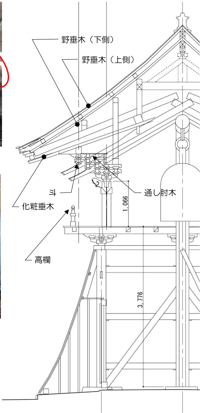
図1 現状梁間断面図
