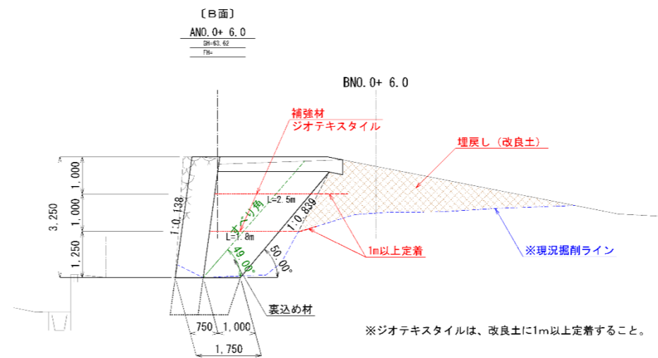
現代工法 (案) 【中門北側石垣】
